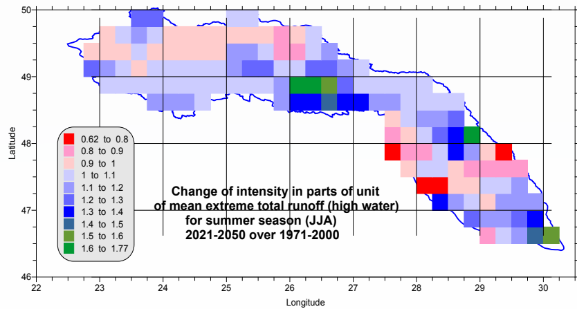
Рисунок 6.16. Проекция изменения интенсивности паводков (отношение будущего к базовому периоду) в бассейне Днестра на период 2021-2050 гг.
