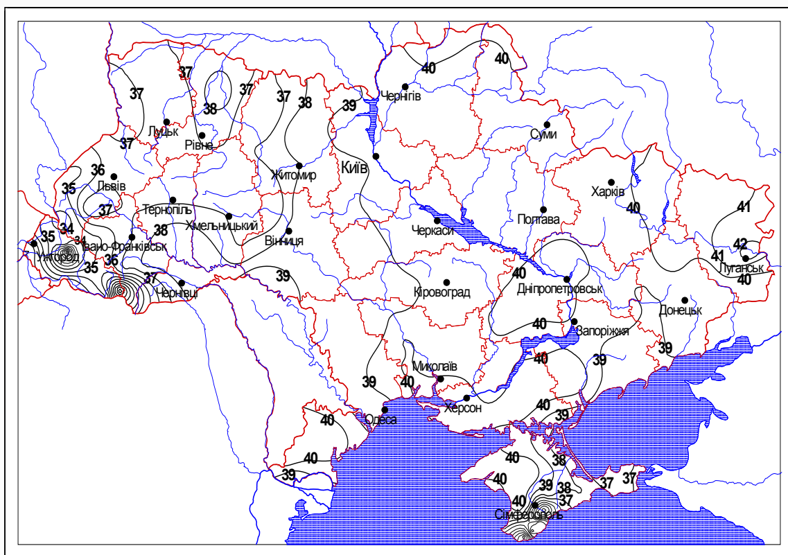
Рисунок 2.5. Абсолютный максимум температуры воздуха ( ^{\circ}\text{C} ). Год
